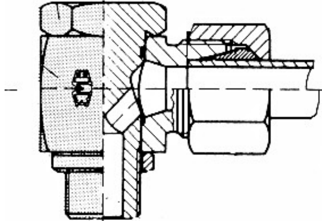
SBE – úhlové nastavitelné šroubení s měkkým těsněním
