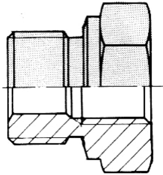
RI - redukce
