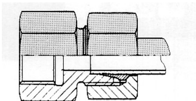
Ai – přímé hrdlo
