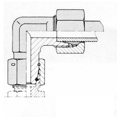
VBDKO – úhlové stavitelné šroubení s O-kroužkem
