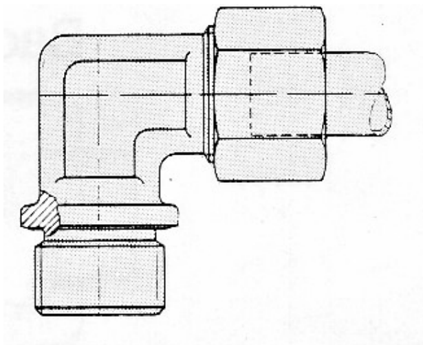
B – úhlové hrdlo
