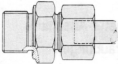
A - přímé hrdlo
