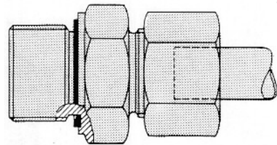
A...-/wd - přímé hrdlo s měkkým těsněním
