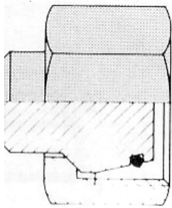
STO - zátka s O-kroužkem
