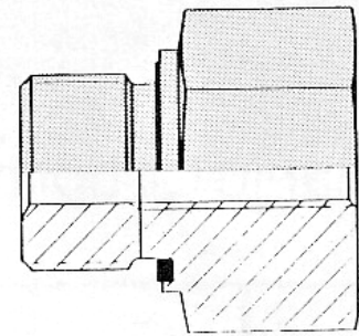
RI...-/WD - redukce
