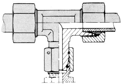
VCDKO – úhlové stavitelné šroubení s O-kroužkem
