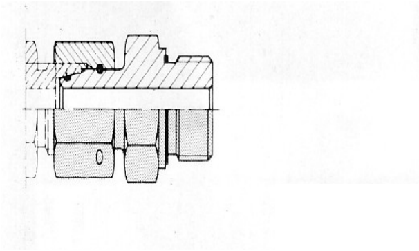
VADKO – stavitelné šroubení s O-kroužkem
