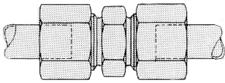
E – spojka přímá
