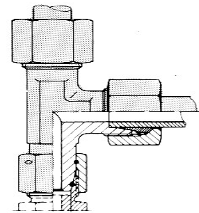
VBDKO – úhlové stavitelné šroubení s O-kroužkem
